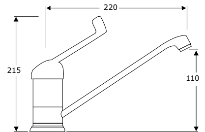
MONOMANDO FREGADERO GERONTOLÓGICO Ref. 65401
